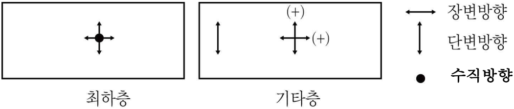
[별도 6] 일반 직사각형 건축물의 지진가속도감지기 설치 위치 및 계측 성분(제15조 관련)
